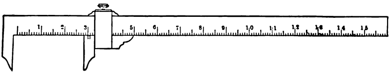
FIG. 46.—Steel Increment Calipers.
